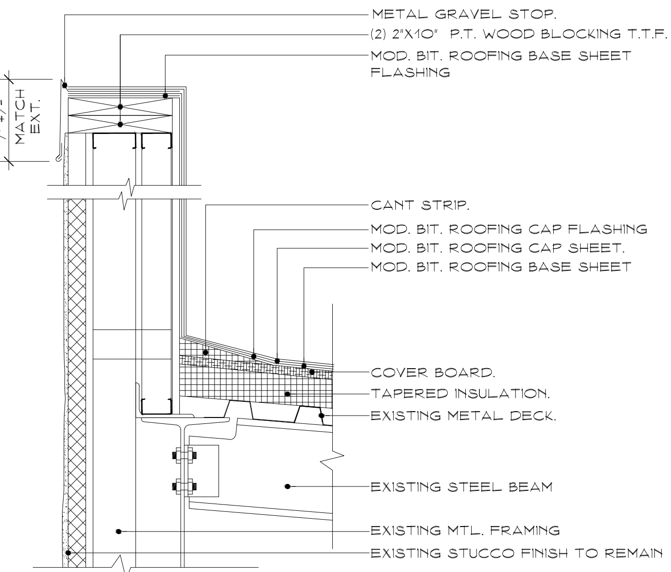
DETAIL @ ROOF EDGE SCALE: 1/2" = 1'-0"
